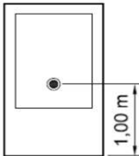
<라. 큰 유리판이 있거나 전체가 유리인 문>
