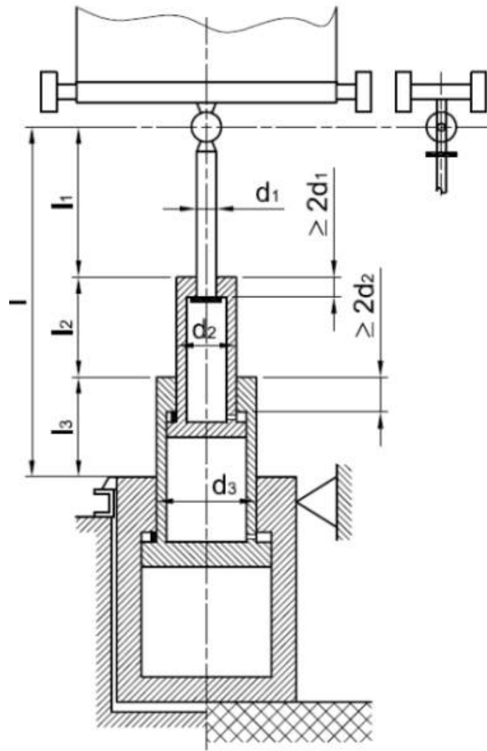
[ 그림 XI.6 - 외부 안내 없는 다단 잭 ]
