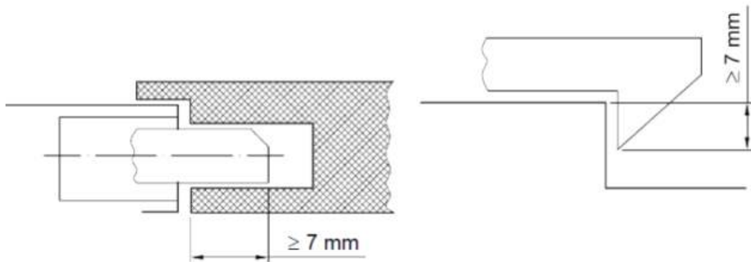
[ 그림 12. 잠금 부품의 예시 ]
