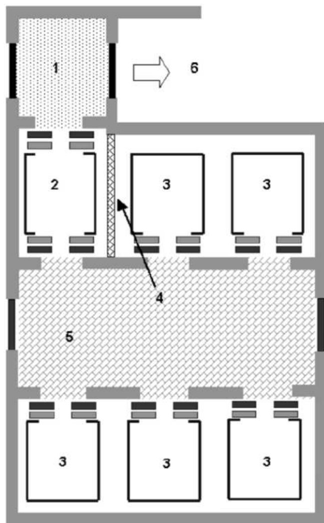
[ 그림 24.3 - 다수의 승강로에 있는 이중 출입 소방구조용 엘리베이터 및 방화 구획된 로비의 배치도 ]
