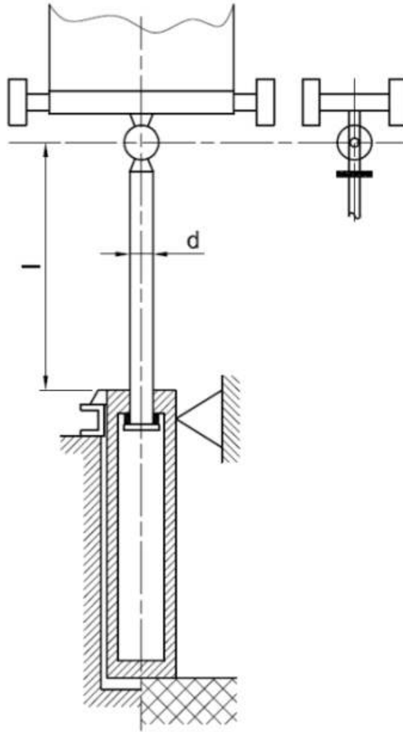
[ 그림 XI.5 - 단 작동 잵 ]
