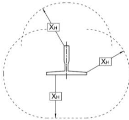
[ 그림 6. 주행안내 레일 주변의 수평 거리 X_H ]
