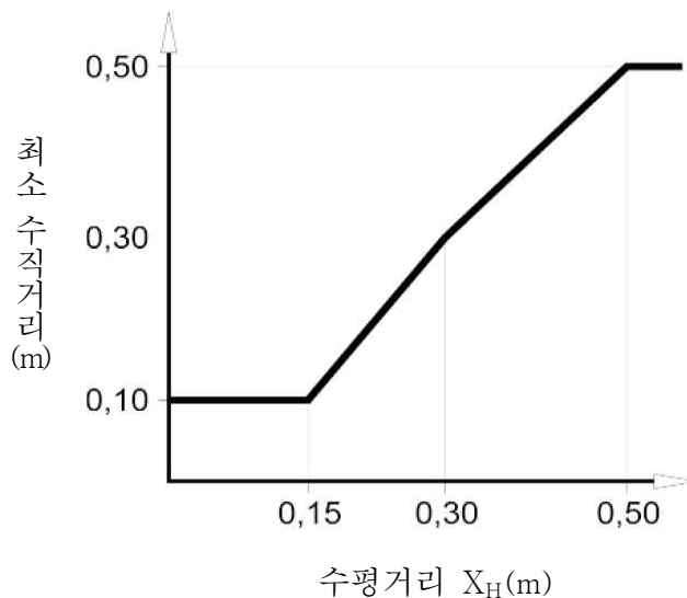
[ 그림 7. 카 프레임 부분, 추락방지안전장치, 가이드 슈/롤러, 멈춤 쇠 장치의 최소 수직 거리 ]
