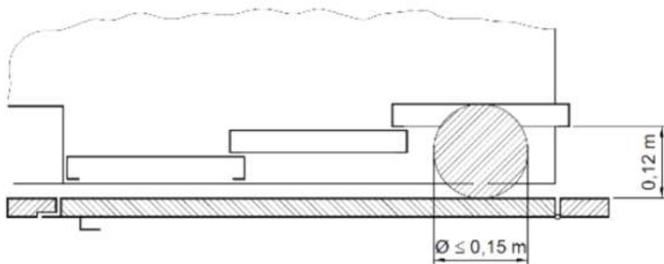
[ 그림 9. 경첩이 있는 승강장문과 수평 개폐식 카문의 조합 ]
