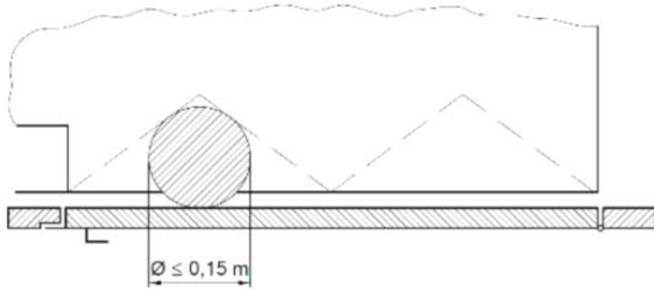
[ 그림 8. 경첩이 있는 승강장문과 접히는 카문의 조합 ]
