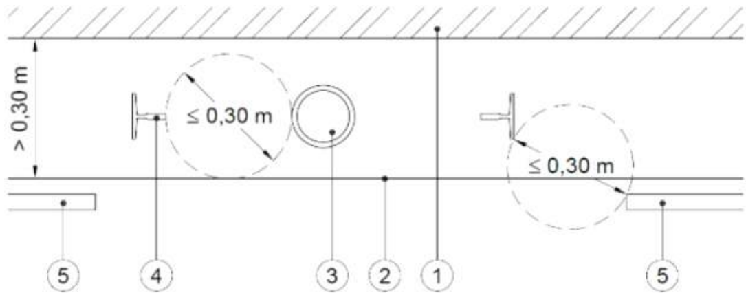
[ 그림 15. 추락 보호 부품의 예(전기식 엘리베이터)]
