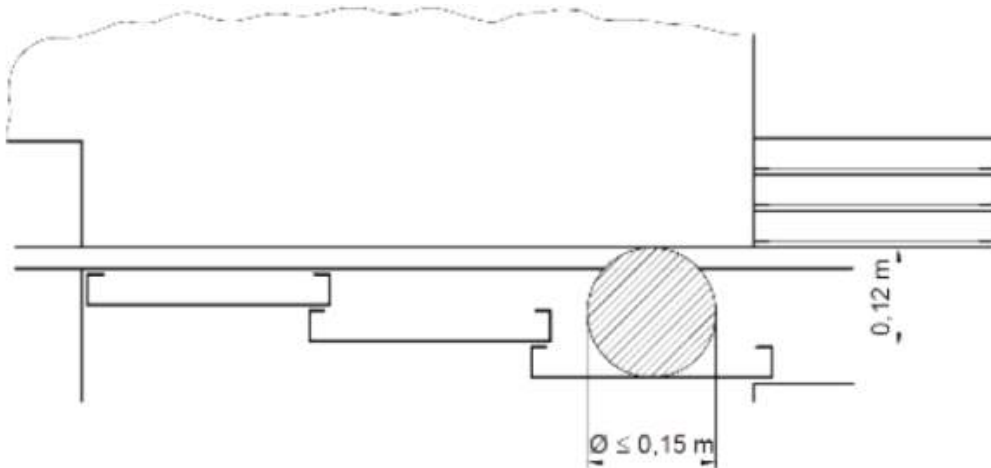
[ 그림 10. 기계적으로 연동되지 않은 수평 개폐식 승강장문과 카문의 조합 ]
