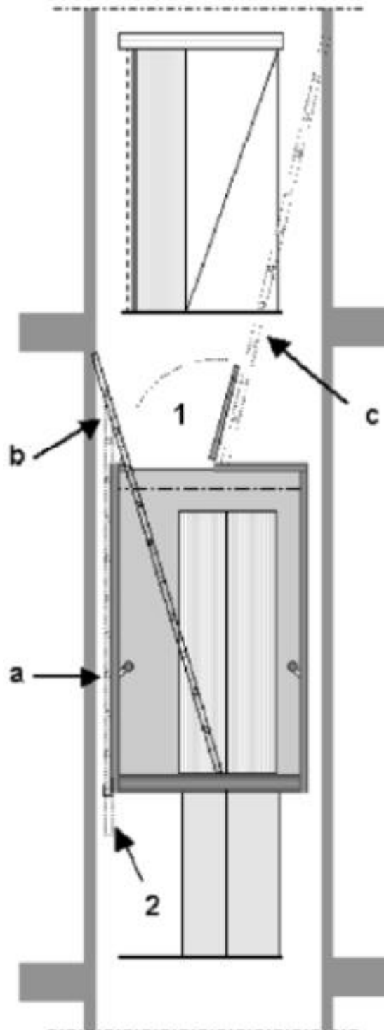
[ 그림 27.1 - 카에 부착된 휴대용 사다리를 이용하여 승강로 밖으로 구출 ]
