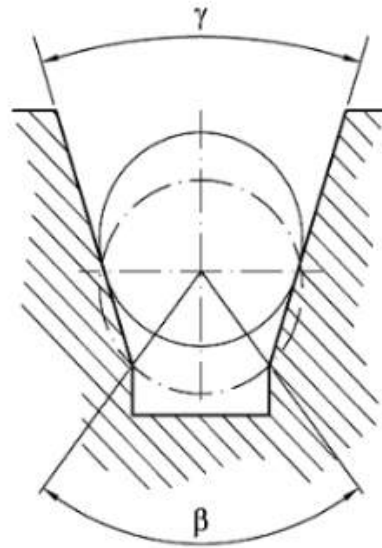
[ 그림 IX.2 V-홈 ]
