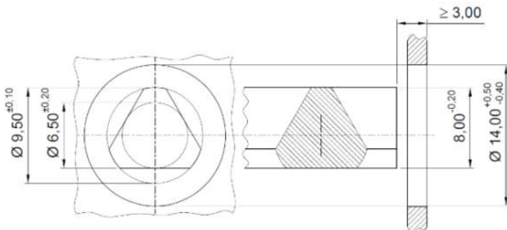
[ 그림 13. 비상잠금해제를 위한 삼각열쇠 구멍 ]
