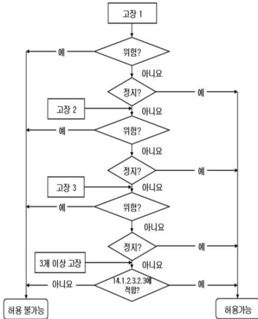
[ 그림 21 - 안전 회로 평가를 위한 순서도 ]
