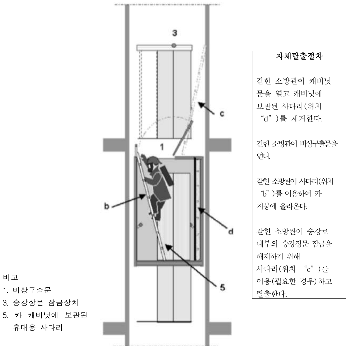
[ 그림 27.3 - 카 내부 캐비닛에 보관된 휴대용 사다리를 이용한 자체 탈출 ]
