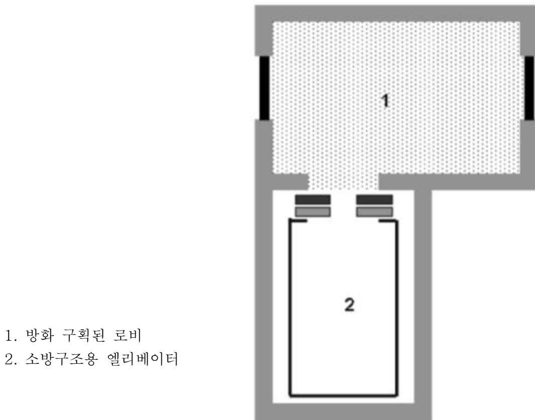
[ 그림 24.1 - 단독 소방구조용 엘리베이터 및 방화 구획된 로비의 배치도 ]
