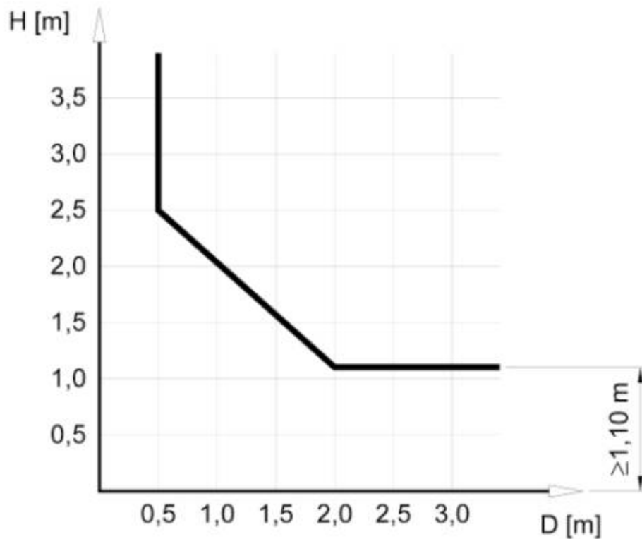
[ 그림 2. 반 밀폐식 승강로 - 거리 ]
