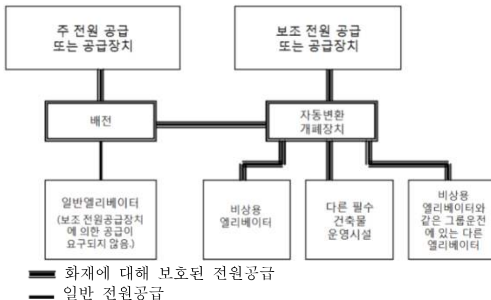
[ 그림 29 - 소방구조용 엘리베이터의 전원공급에 대한 예시 ]
