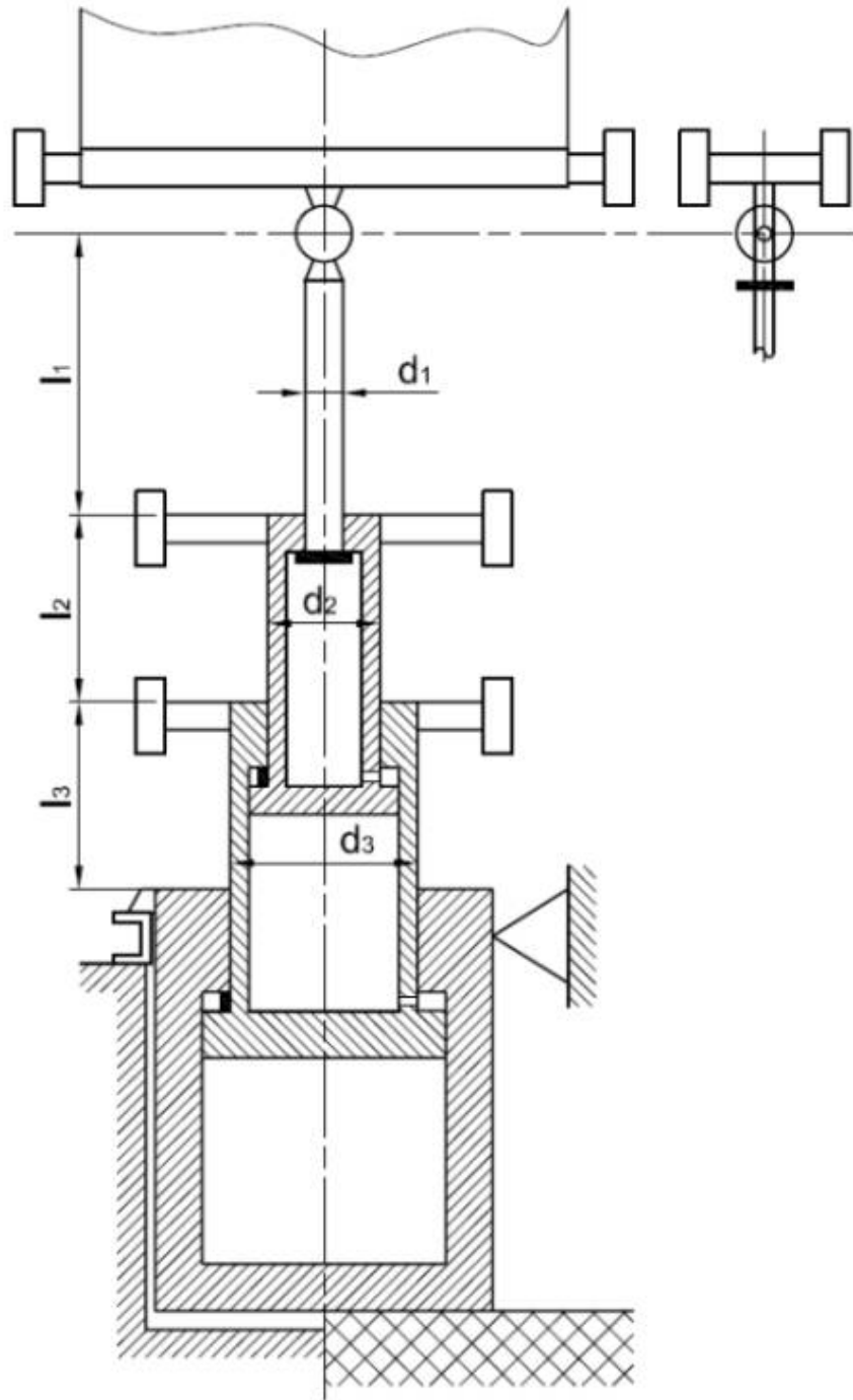
[ 그림 XI.7 - 외부 안내 있는 다단 잭 ]
