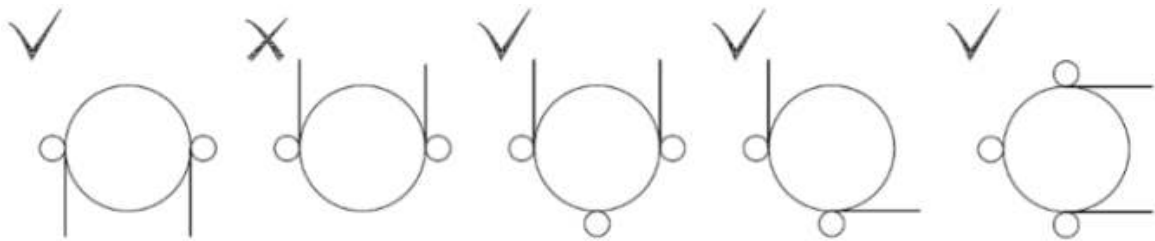
[ 그림 19. 로프 고정장치(retainer)의 배치 예시 ]
