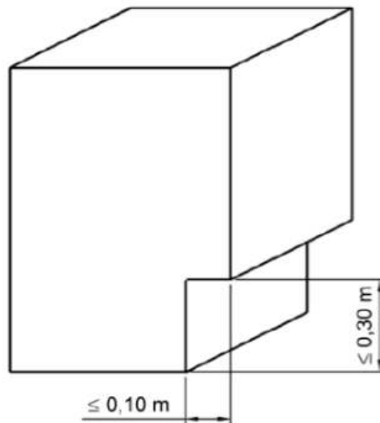
[ 그림 4. - 피난공간 축소의 최대 크기 ]
