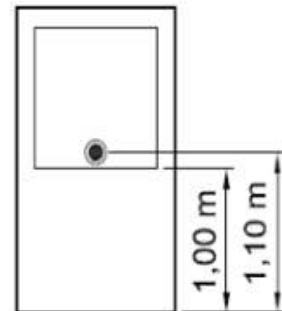
<바. 유리판이 1m 위에 있는 문>
