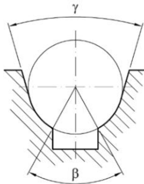
[ 그림 IX.1 반원 언더컷 홈 ]
