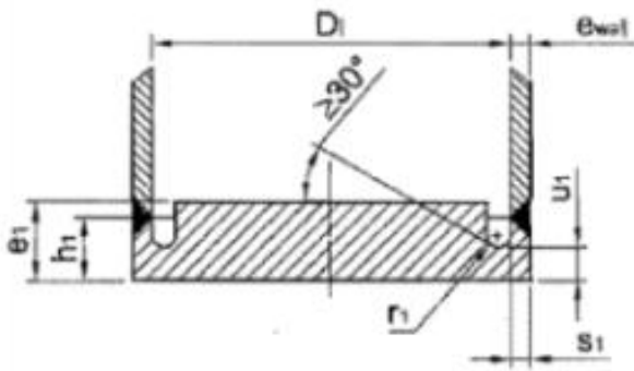
[ 그림 XI.2 - 릴리빙 홈을 가진 편평한 기초 ]
