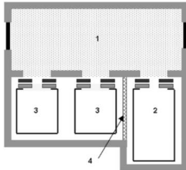
[ 그림 24.2 - 다수의 승강로에 있는 소방구조용 엘리베이터 및 방화 구획된 로비의 배치도 ]
