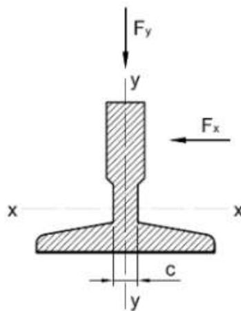
[ 그림 VIII.1 - 주행안내 레일의 축 ]
